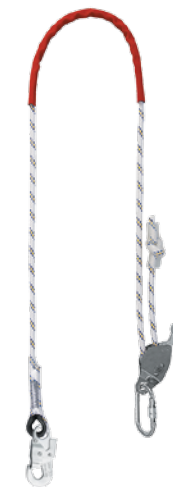
PROT 22 urządzenie do ustalania pozycji przy pracy o dł. 2 m z zatrzaśnikami AZ 002 i AZ 011
